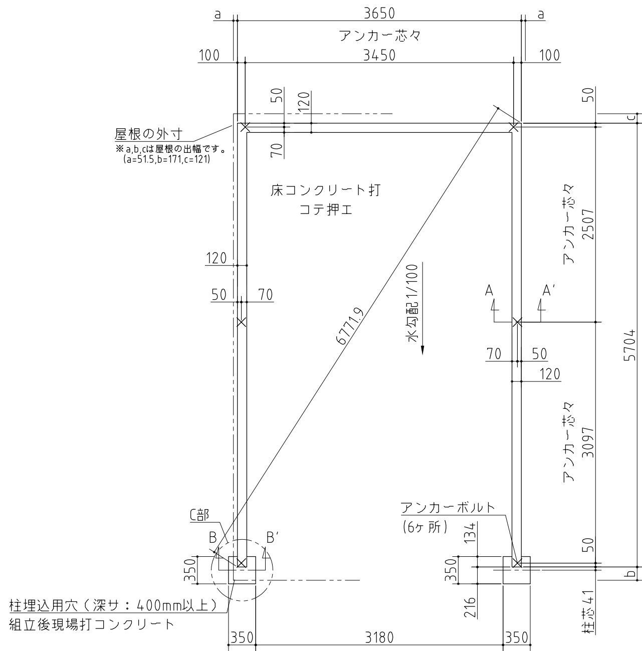
基礎詳細図 S=1/20
